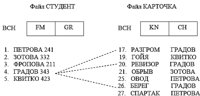
Рис. 35. Записи файлов (один-ко-многим)
