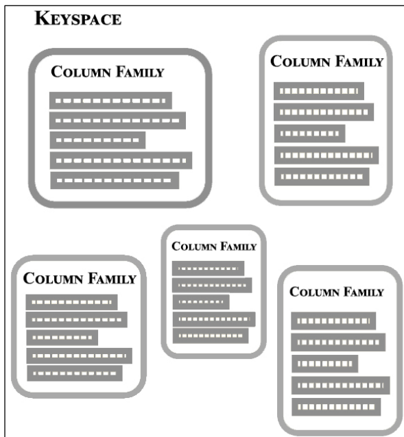
Рис. 25. Пространство ключей, содержащее семейства столбцов
