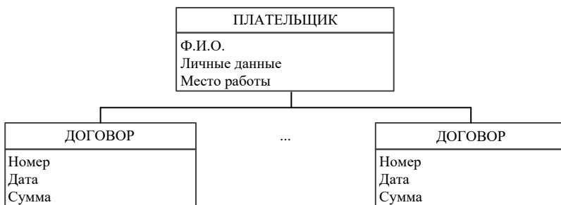
Рис. 16. Дополнительное групповое отношение студент — договор — плательщик
