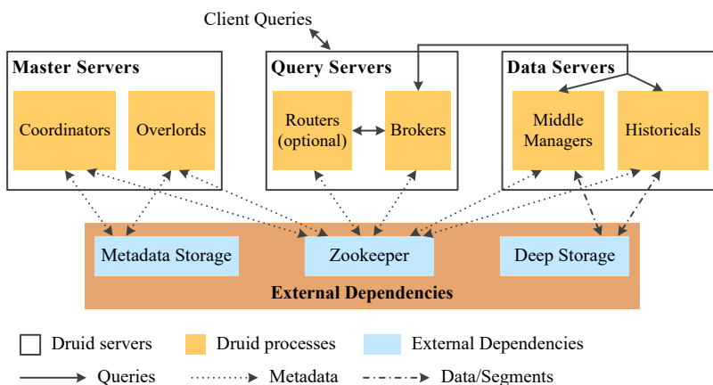
Рис. 29. Архитектура Apache Druid
