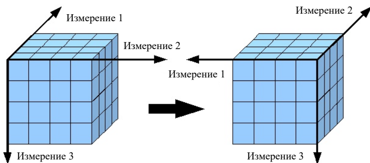
Рис. 3. Операции OLAP: вращение
