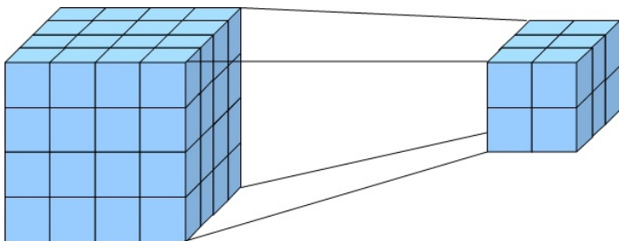
Рис. 5. Операции OLAP: консолидация
