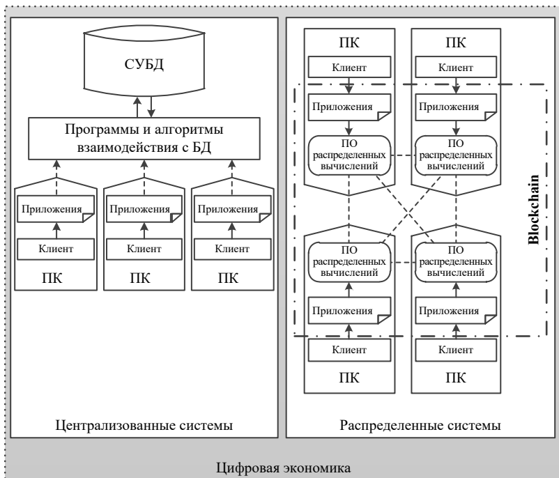
Рис. 23. Роль технологии Blockchain в цифровой экономике
