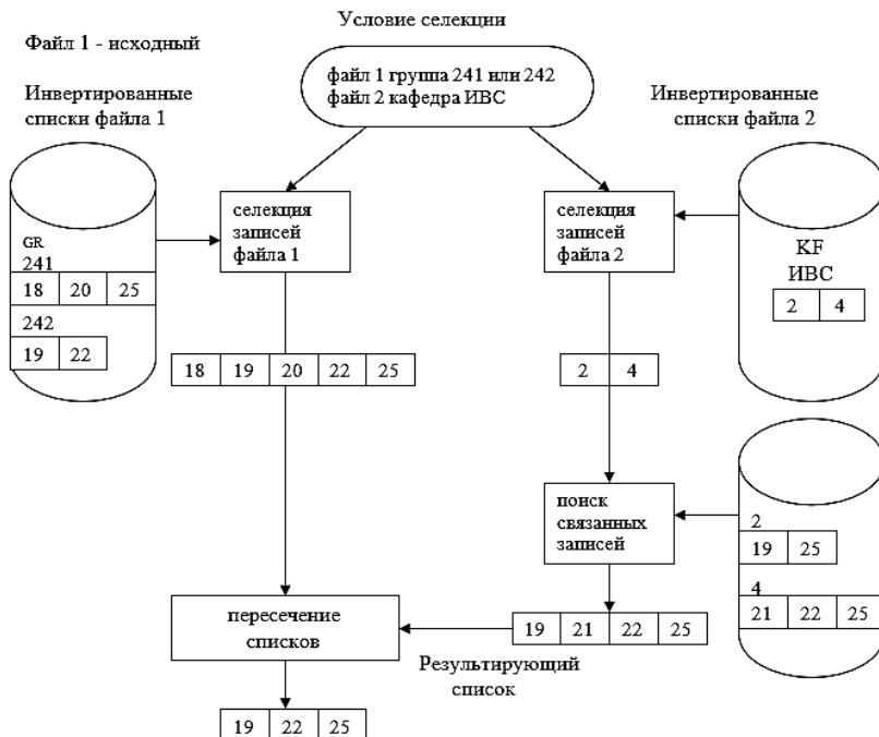
Рис. 43. Ассоциативный поиск записей в связанных файлах
