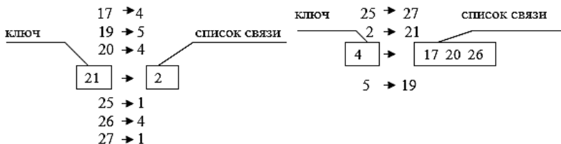
Рис. 37. Списки связи с ключами (один-ко-многим)
