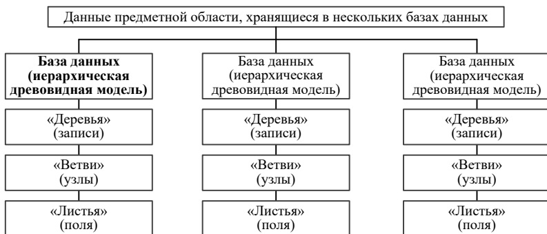
Рис. 12. Компоненты баз данных, основанных на иерархической модели
