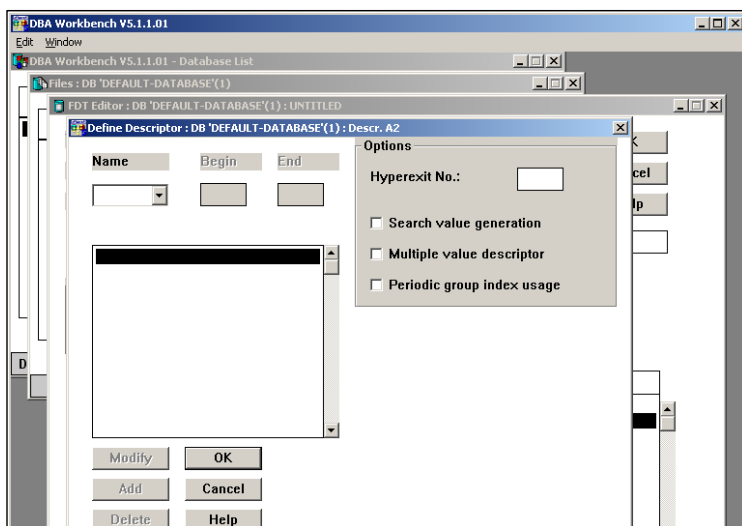
Рис. 74. Определение синтаксиса гипердескриптора
