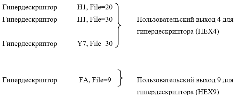
Рис. 73. Гипердескриптор и пользовательские выходы
