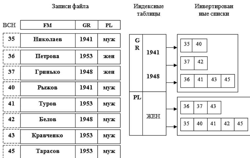
Рис. 33. Записи файла и инвертированные списки до модификации файла
