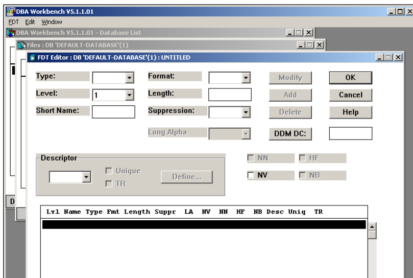
Рис. 65. Создание записи при помощи редактора FDT
