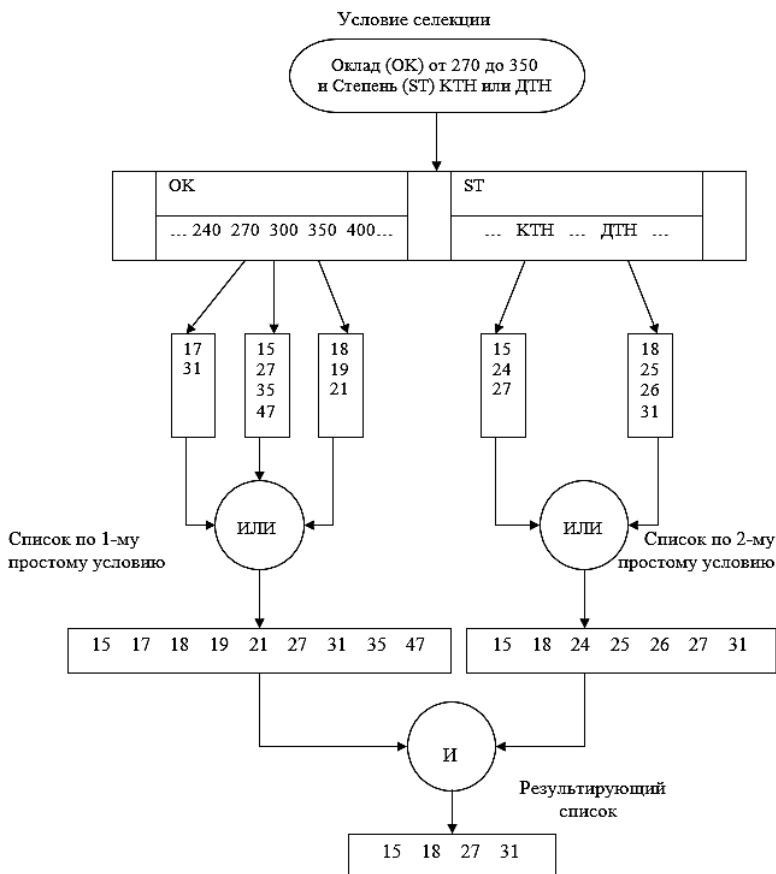
Рис. 42. Ассоциативный поиск записей файла
