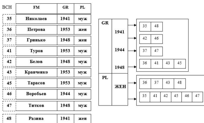
Рис. 34. Записи файла и инвертированные списки после модификации файла
