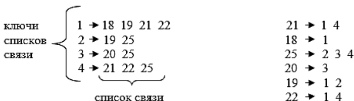
Рис. 40. Списки связи с ключами (многие-ко-многим)
