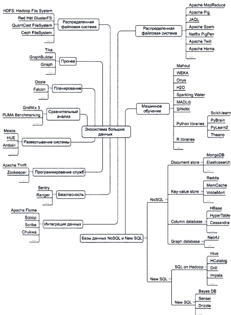
Рис. 11. Технологии больших данных по основным категориям [10, с. 29]
