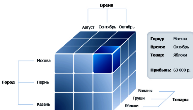
Рис. 1. Пример трехмерного подмножества структуры куба данных 1
