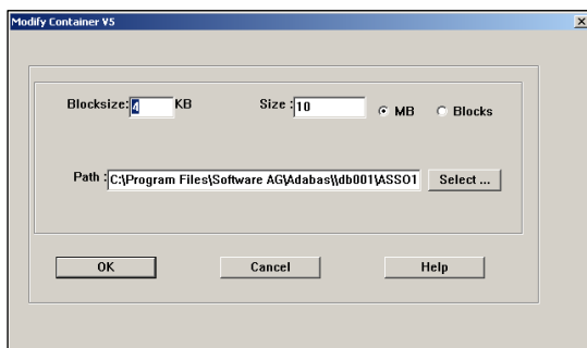
Рис. 51. Изменение параметров файлов структуры
