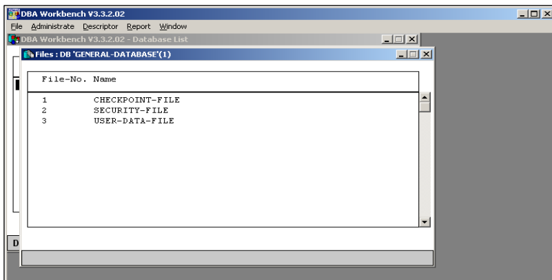
Рис. 60. Список уже существующих файлов БД
