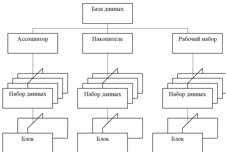
Рис. 44. Структура базы данных
